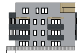
PROČELJE ZAPAD
