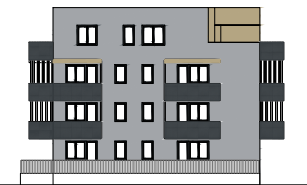
PROČELJE ZAPAD
